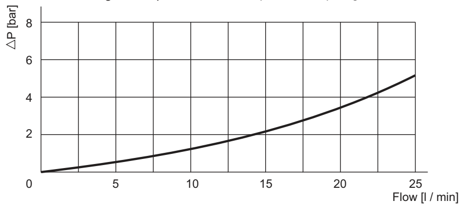
Diagramma perdita di carico - pressure drop diagram
